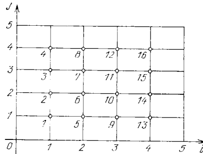
Рис. 14. Одномерная нумерация двумерного массива
