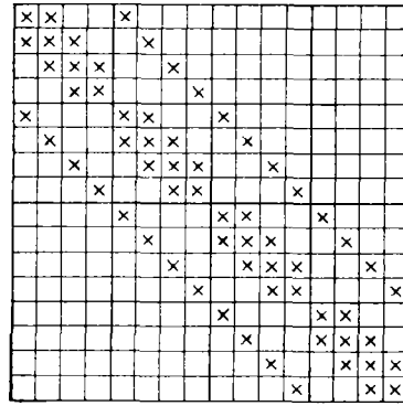
Рис. 15. Структура матрицы системы (5) для N=5
